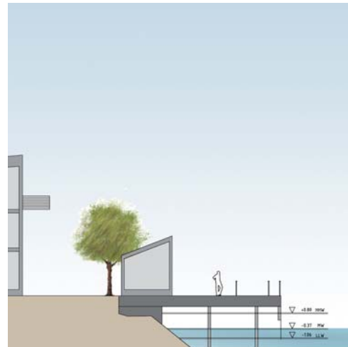
Sektion 2C-2C genom kaj och kioskbbyggnad nedanför bruket.
